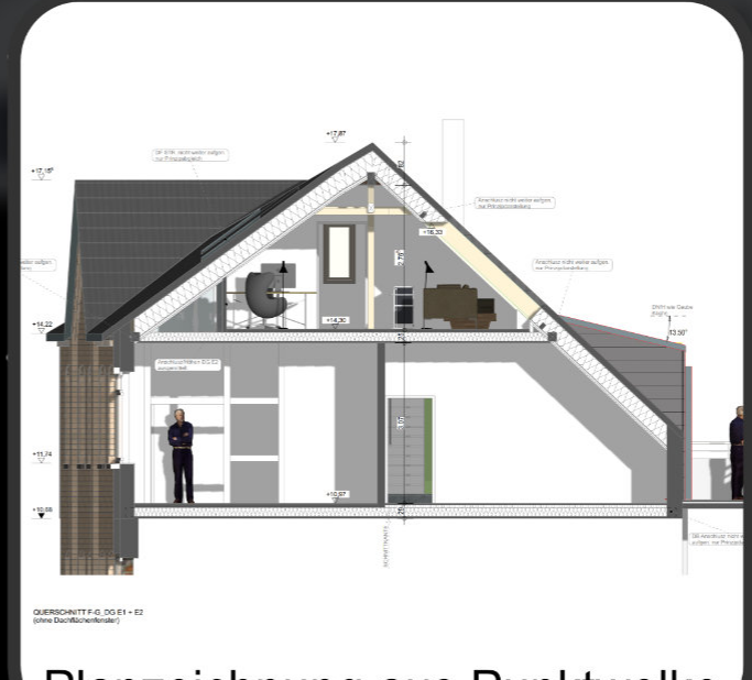
Planzeichnung aus Punktwolke
